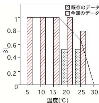
図-4 水温の選好曲線
