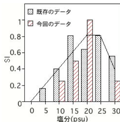
図-3 塩分の選好曲線
