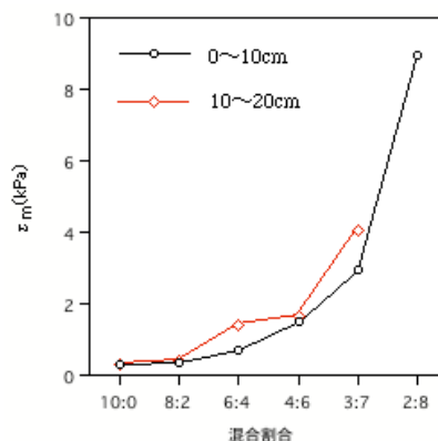
図-5 底泥表層の剪断強度 d/D= 1.03 1.53 0.7 0.8 0.5 0
