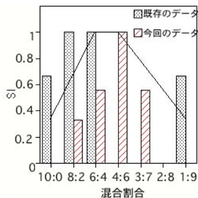
図-2 混合割合の選好曲線
