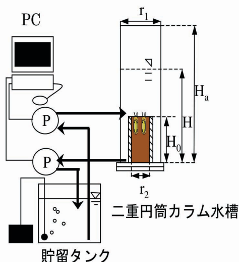
図-1 室内生息実験装置
