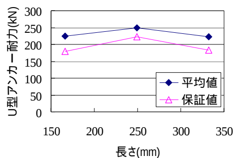
図-6 U 型アンカー長さの影響
