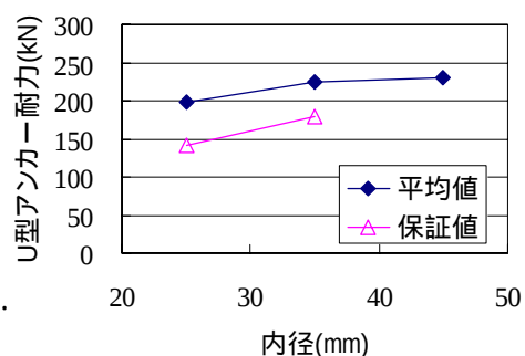
図-5 U 型アンカー内径の影響
