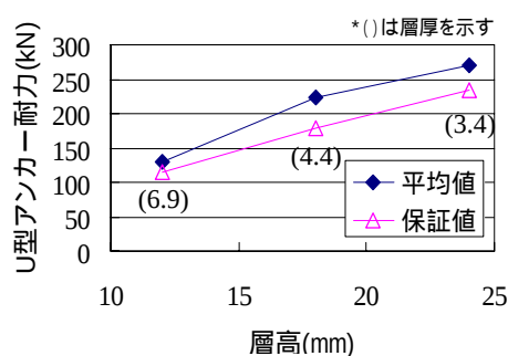
図-7 層高（層厚）の影響
