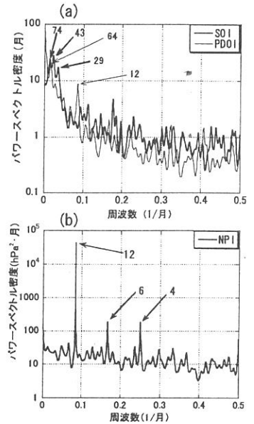
図-4 パワースペクトル密度
