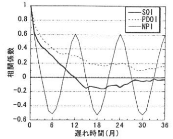
図-3 各指標の自己相関関数
