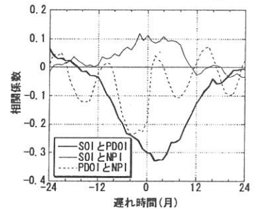
図-5 各指標間の相互相関関数
