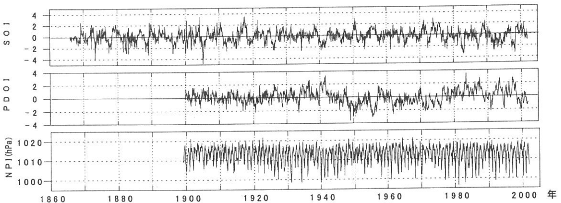
図-1 各大気海洋指標の時系列
