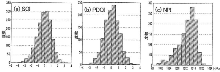
図-2 各大気海洋指標のヒストグラム
