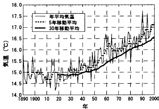
図-1 福岡市年平均気温時系列
