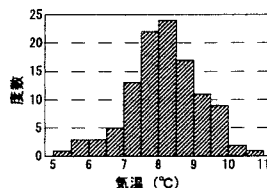
図-3 トレンド除去後月平均気温ヒストグラム(3月)
