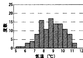
図-2 月平均気温ヒストグラム(3月)
