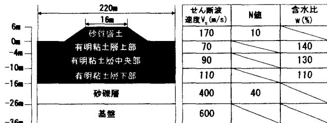
図-3 モデル地盤
