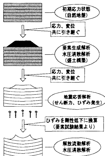
図-1 残留変形解析のフロー
