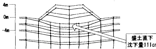
図-6 盛土付近の地震時残留変形(塩分溶脱後)
