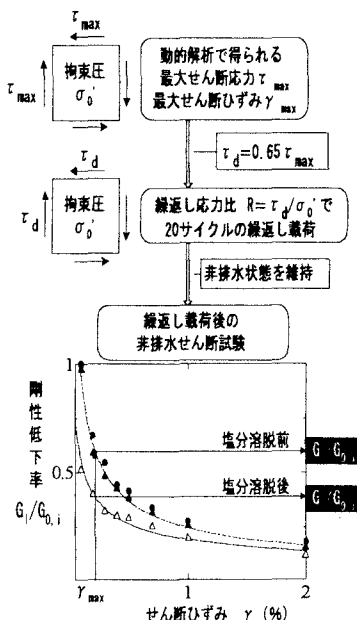
図2 剛性低下率の算出方法
