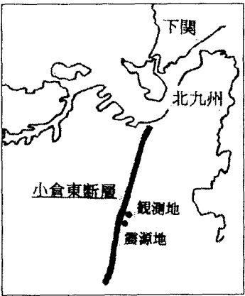
図-1 小倉東断層の位置
