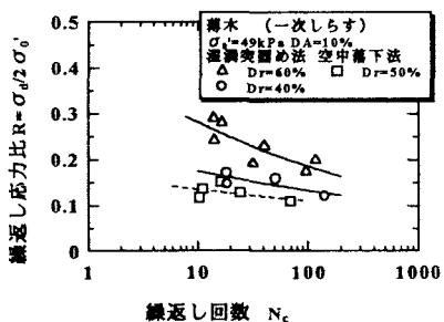
図4 RとNcの関係(薄木)
