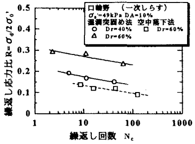
図3 RとNcの関係(口輪野)
