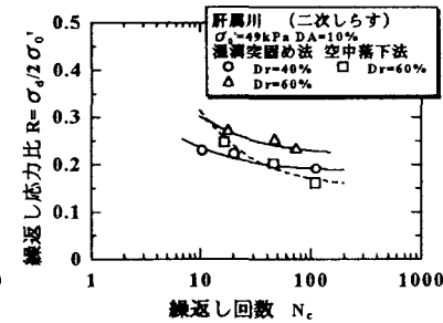
図6 RとNcの関係(肝属川)
