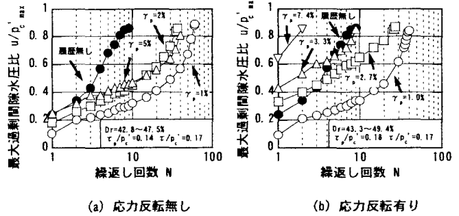
図-4 繰返し回数と最大過剰間隙水圧比の関係
