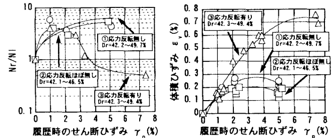
図-6 \gamma_p と N_r/N_l の関係
