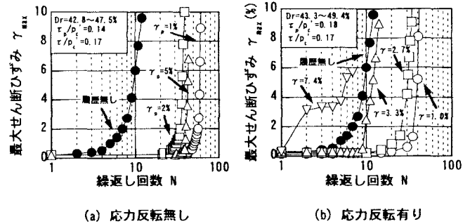
図-5 繰返し回数と最大せん断ひずみの関係
