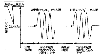
図-1 実験模式図
