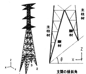
図-2 基部支柱材の番号及び支間の傾斜角
