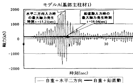
図-5 地震波の入力方向による応答軸力時刻歴の比較
