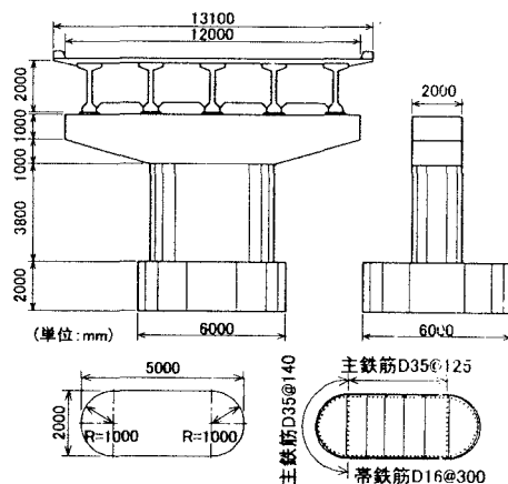
図-2 一般構造図
