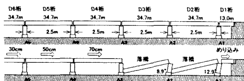
図-1 長庚橋損傷状況図
