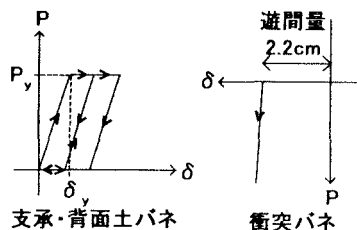
図-4 各バネモデル図
