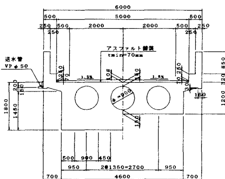
図-1 断面図
