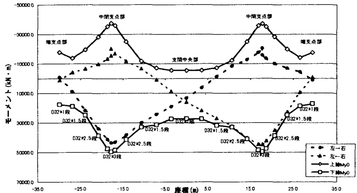
図-4 上部曲げ耐力照査結果(橋軸方向)
