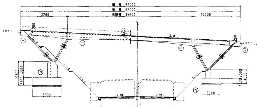
図-2 側面図
