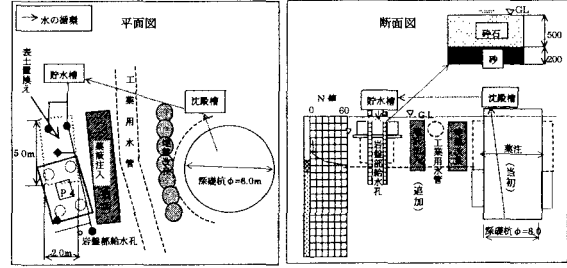
図-4 復水工法計画図
