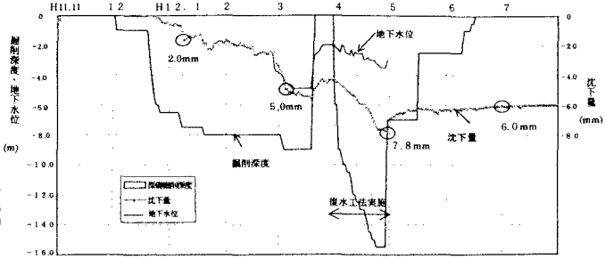
図-3 掘削-沈下相関図
