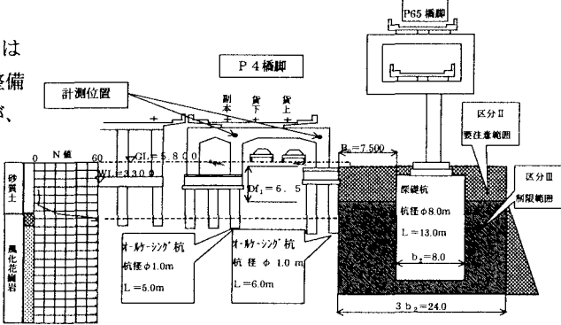
図－2 断面図
