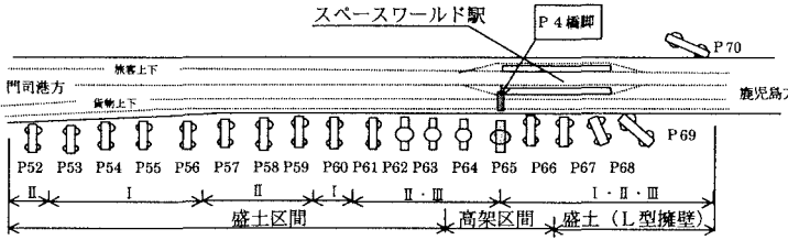
図－1 平面図
