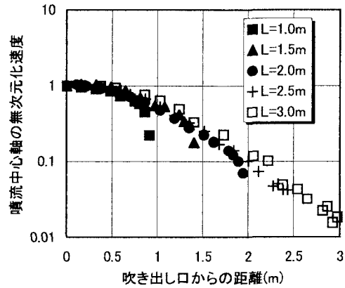
図 3 噴流の中心軸上の速度と風管距離 L の関係( D=0.15\text{m} )
