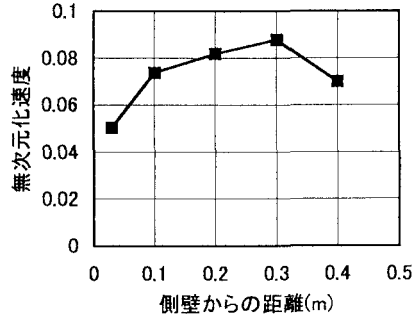
図 5 切羽面近傍 0.01\text{m} における無次元化速度側壁からの距離の関係( L=2.0\text{m} , D=0.15\text{m} )
