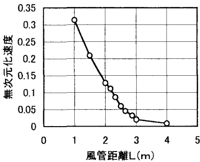
図 4 切羽面中心から 0.01\text{m} 離れた点における無次元風速と風管距離 L の関係( D=0.2\text{m} )
