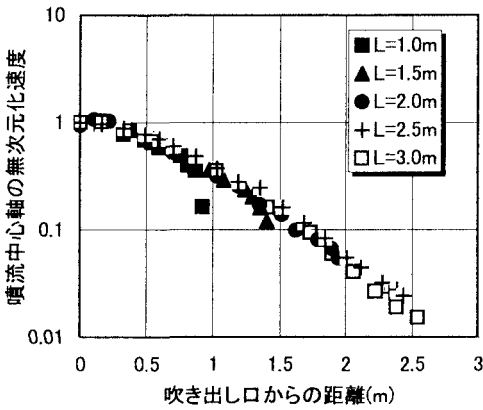
図 2 噴流の中心軸上の速度と風管距離 L の関係( D=0.1\text{m} )
