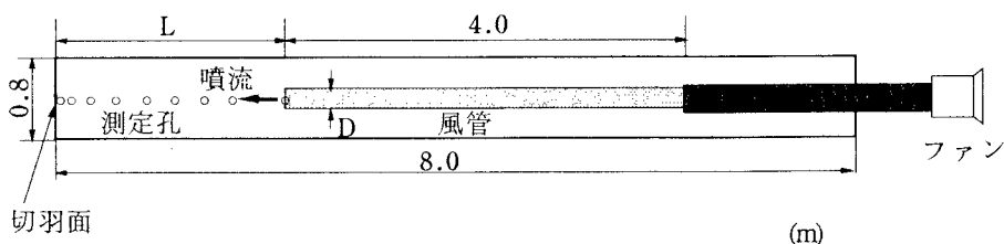
図 1 掘進切羽模型の概略図
