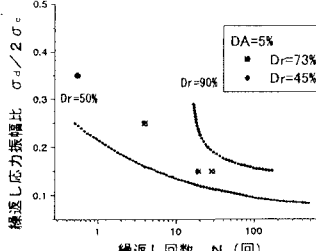
図-7 繰返し応力比と繰返し回数の関係
