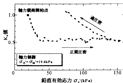
図 1 K_o 値と \sigma_v' の関係(軸力制御)
