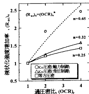
図6 (R_{oc})_v と (OCR)_v の関係
