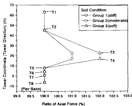
図-5 主塔の最大軸力
