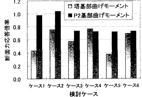
図-5 免震ケースによる応答断面力比較
