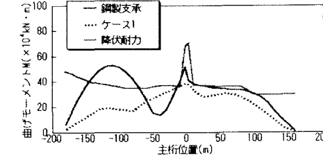
図-6 主桁面外応答曲げモーメント
