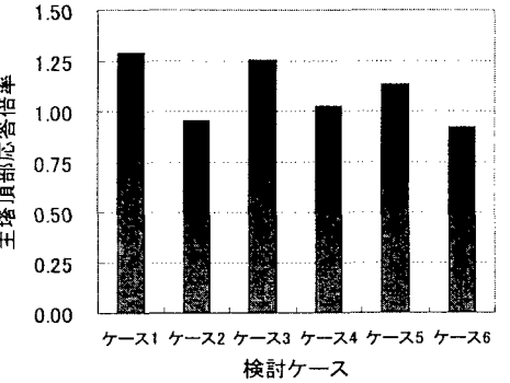
図-4 免震ケースによる塔頂変位比較
