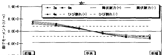
図-9 橋軸直角方向させた場合におけるP1橋脚横梁部の曲げモーメント M_x 最大値分布
