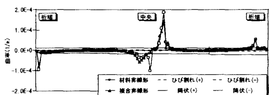
図-10 複合非線形解析と材料非線形解析における応答曲率の比較 (6m鉛直方向変位時)
