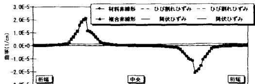
図-11 複合非線形解析と材料非線形解析における応答曲率の比較 (6m橋軸直角方向変位時)
