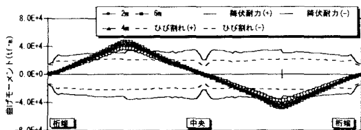
図-7 橋軸直角方向変位させた場合における主桁の曲げモーメント M_x 最大値分布
