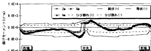
図-4 鉛直方向変位させた場合における主桁の曲げモーメント M_x 最大値分布
