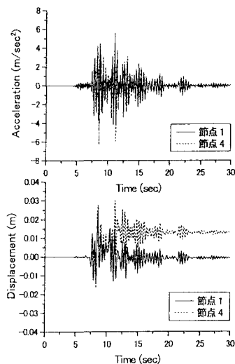
図-2 時刻歴応答
