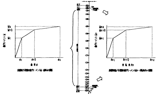
図-4 下部工モデル
