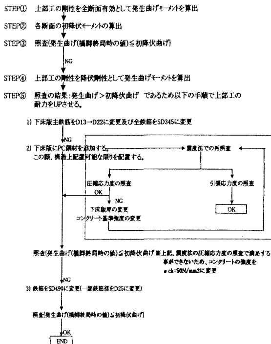
図-2 解析フロー
