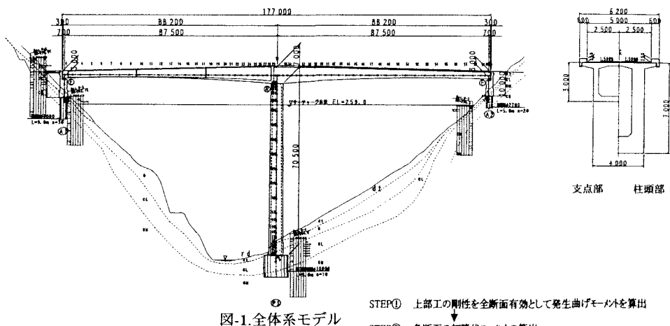
図-1.全体系モデル
