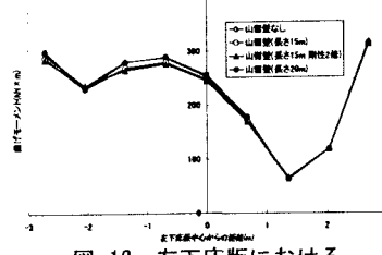
図-12 左下床版における最大曲げモーメント
