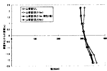
図-4 左側壁における最大軸力
