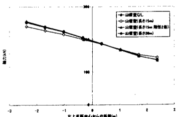
図-7 左上床版における最大軸力
