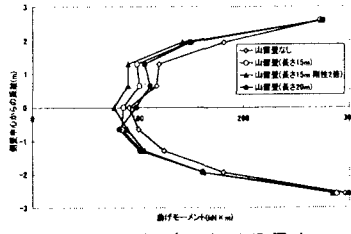
図-6 左側壁における最大曲げモーメント
