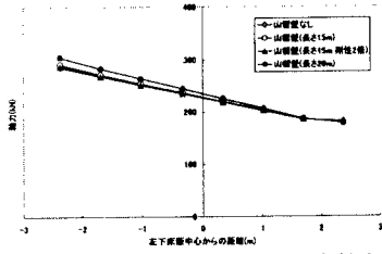
図-10 左下床版における最大軸力
