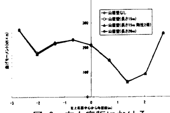
図-9 左上床版における最大曲げモーメント
