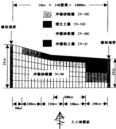
Fig. 2 実地盤モデル (A-A' 断面)
