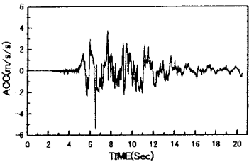
Fig. 3 入力地震波
