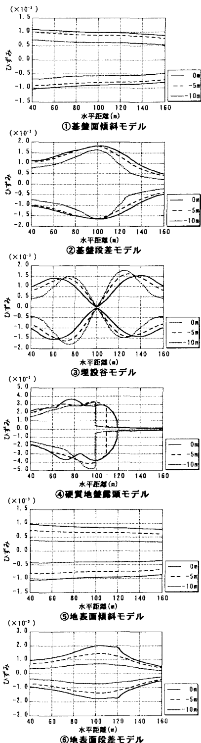
図-2 最大軸ひずみ分布 (引張+, 圧縮-)
