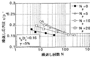
図-5 液状化強度曲線 ( Dr=40\% )
