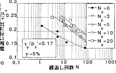
図-6 液状化強度曲線 ( Dr=60\% )
