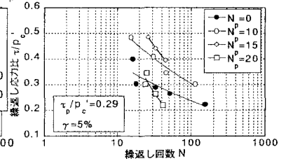
図-7 液状化強度曲線 ( Dr=80\% )
