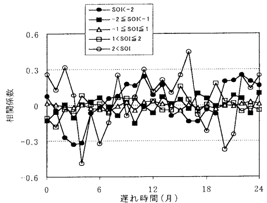
図-3 分類したSOIと福岡市月降水量の相互相関
