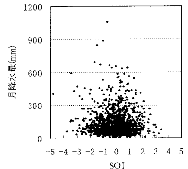
図-4 SOIと4ヶ月後月降水量の散布図
