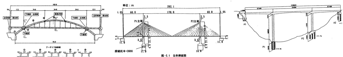
図-1 橋梁概要図
