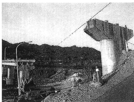
写真-1 P1橋脚の隆起による碑豊橋の落橋
