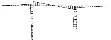
図-10 モーメント図 (面内方向)
