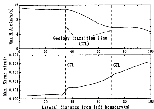
Fig.3 神戸地盤モデルにおける
