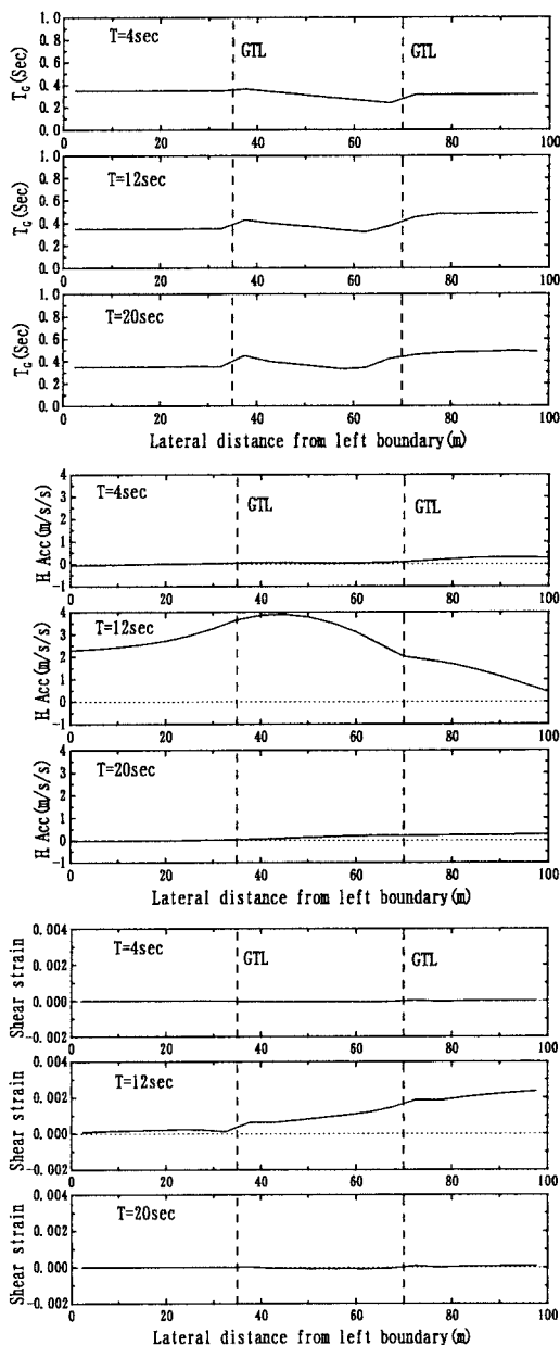
Fig.2 神戸地盤モデルにおける地盤の固有周期・
