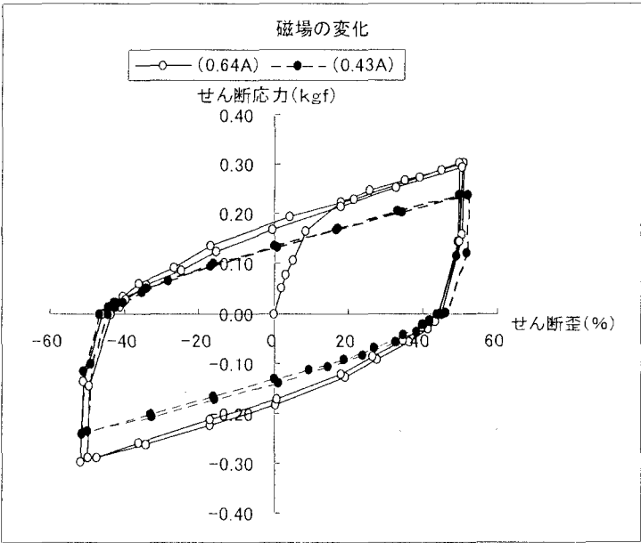
図-2 くり返し変位
