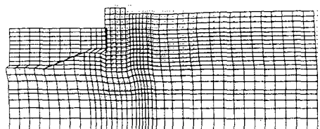
図5 残留変形図(主要部)
