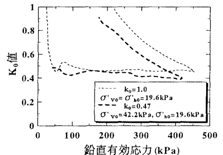
図 2 鉛直有効応力と K 0 値の関係
