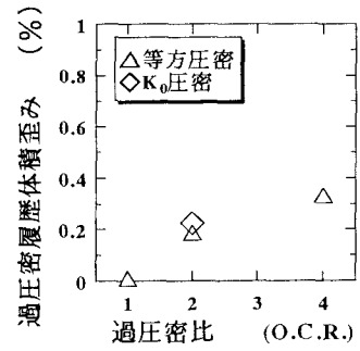
図 6 過圧密履歴体積ひずみと過圧密比の関係
