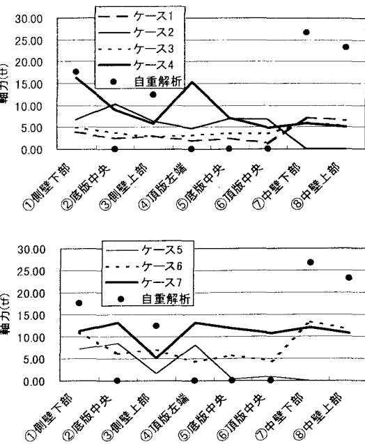
図3 増分断面力比較（軸力）
