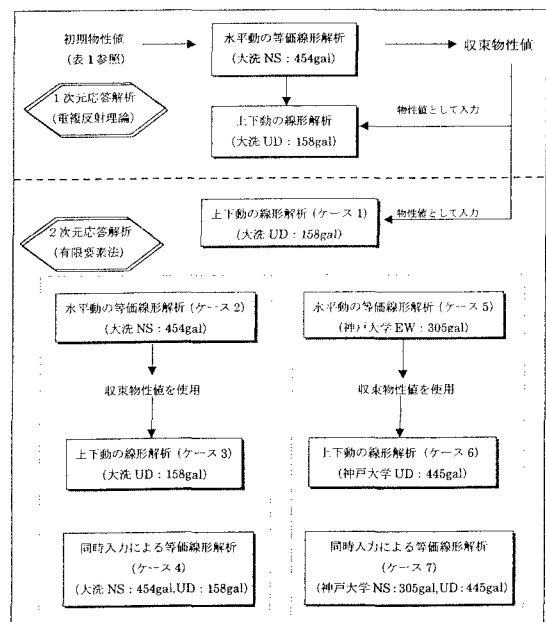
図1 解析フロー
