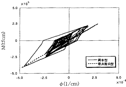
図-3 曲げモーメント-曲率履歴曲線
