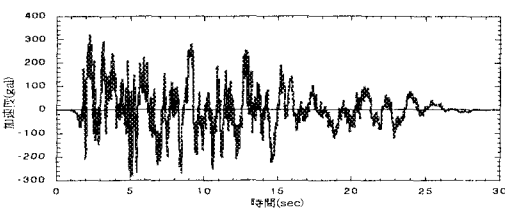
図-2 入力地震動
