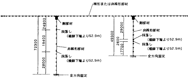
図-1 解析モデル (単位: mm)
