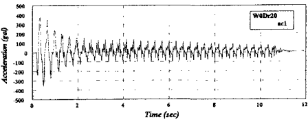
図-2 入力加速度
