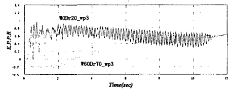
図-6 埋設構造物底面の間隙水圧比時刻歴
