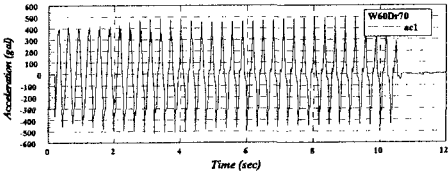
図-3 模型埋設構造物応答加速度
