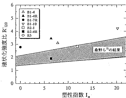
図4 液状化強度比と塑性指数の関係
