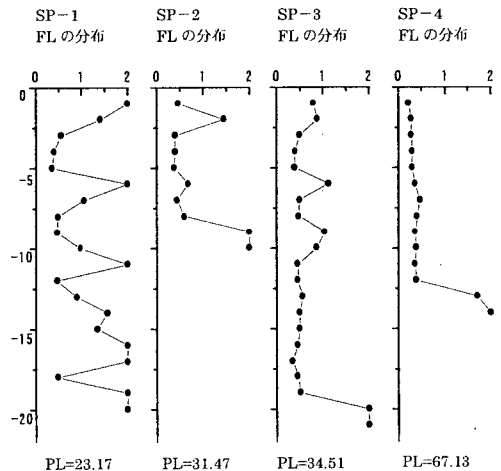
図-5 各地点における液状化判定結果
