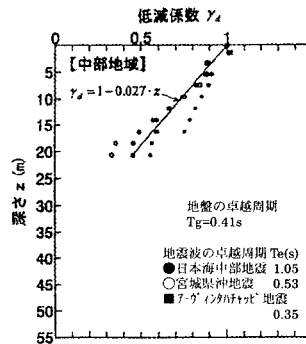
図-1 鹿児島市南部地域の 深さ方向の低減係数
