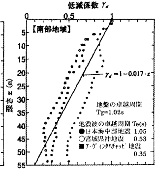
図-2 鹿児島市中部地域の 深さ方向の低減係数
