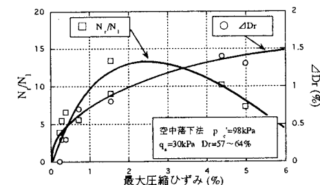
図-8 繰返し履歴時の最大圧縮ひずみと N_r/N_i と \Delta Dr の関係
