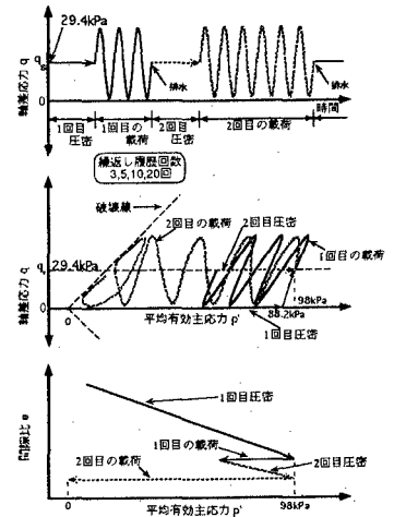
図-1 実験の模式図
