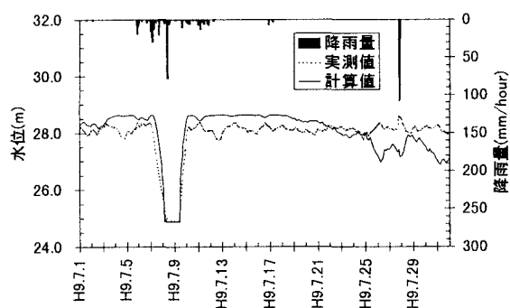
図-3(c) H貯水池水位変化
