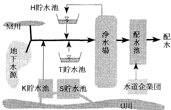
図-1 S町水需給システム概念図
