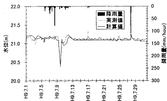
図-3(b) K貯水池水位変化
