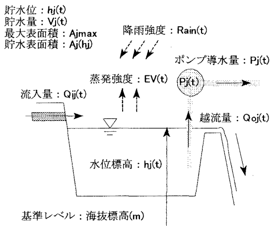
図-2 貯水池の水収支モデル
