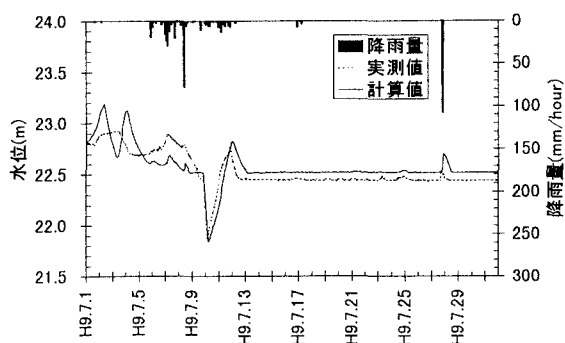
図-3(a) S貯水池水位変化
