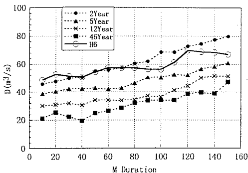
図-4 瀬の下観測点のDDC (1月起点)
