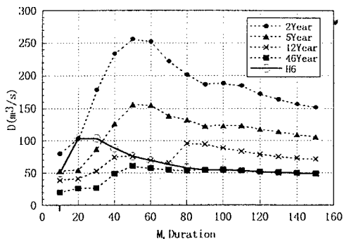
図-5 瀬の下観測点のDDC (6月起点)
