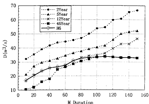
図-3 瀬の下観測点のDDC
