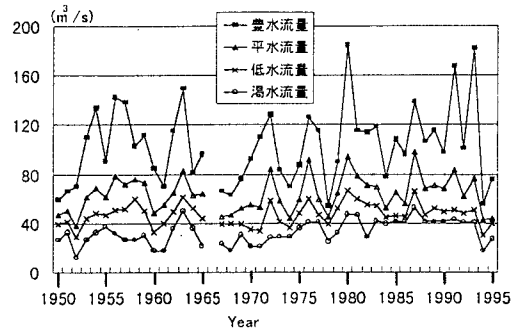
図-2 瀬の下の流量の変動図
