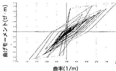
図-10 履歴曲線 (TYPE2)
