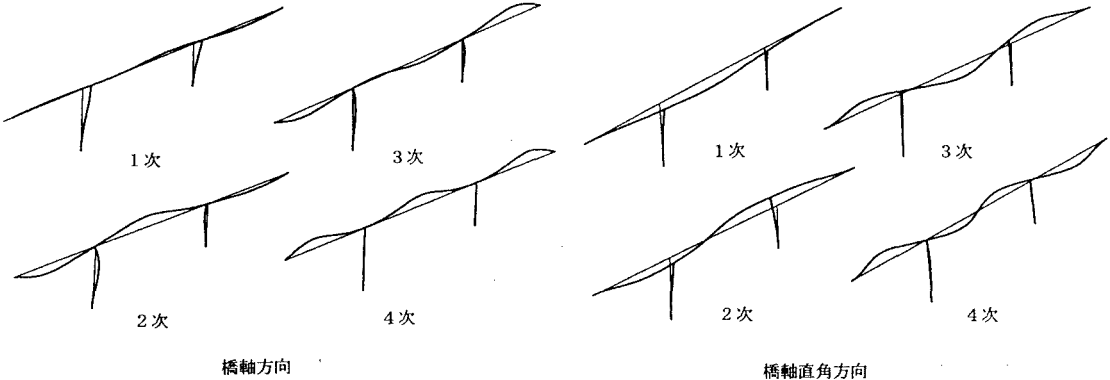
図-2 モード図
