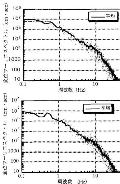
図-1 震源スペクトル(上: 3/26 地震、下: 5/13 地震)
