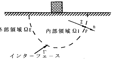
Fig.1 無限領域モデル
