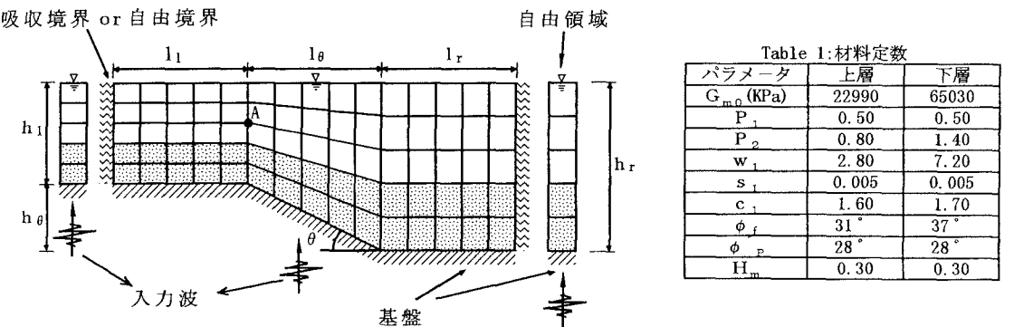
Fig. 2 2次元不整形モデル
