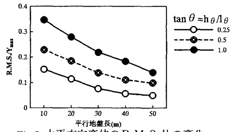
Fig. 5 水平方向変位のR.M.S.比の変化 (吸収境界)
