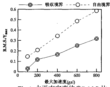
Fig. 4 水平方向変位のR.M.S.比
