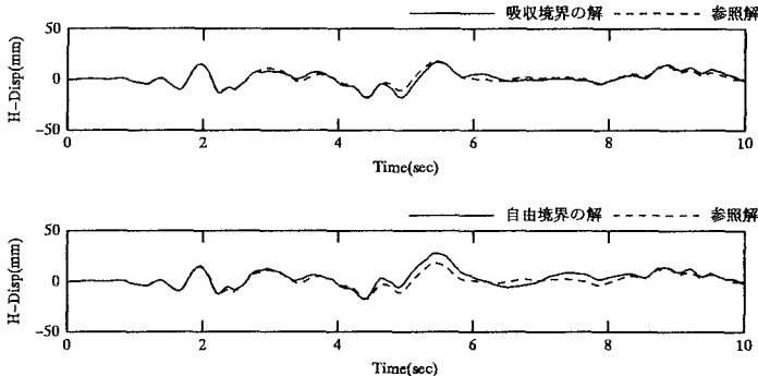
Fig. 3 水平方向変位の応答波形 ( \theta=0.5 , l_1=l_r=50m )
