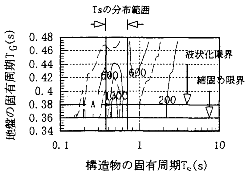
図4 加速度応答スペクトル(単位；cm/s 2 )
