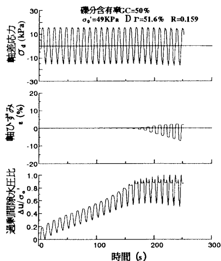
図-5 時刻歴
