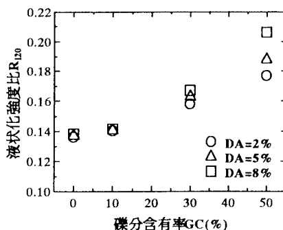
図-6 液状化強度比 R_{120} ～礫分含有率 GC 関係
