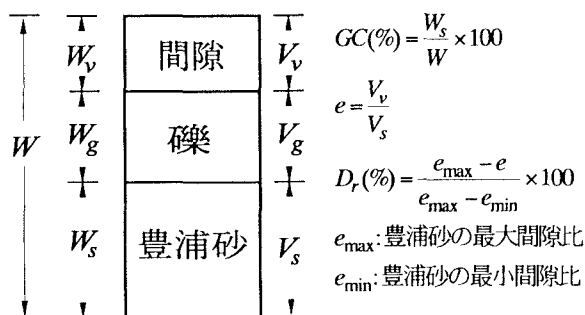
図-1 礫混入時の礫分含有率及び相対密度の説明図
