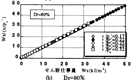
図-4 Ws と Ws/(u/p'_c) の関係
