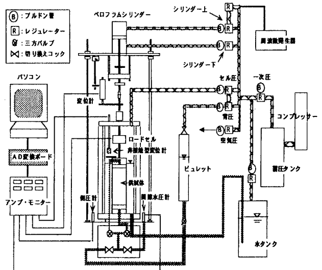
図-1 空圧制御繰返し三軸試験装置配管系統図
