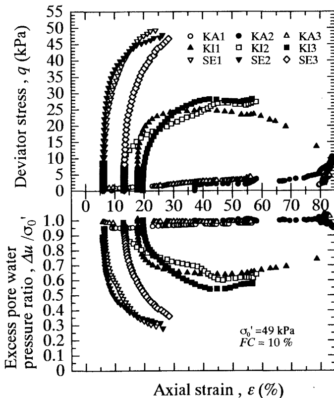
図2 液状化後の q \cdot \Delta u \sim \varepsilon 関係
