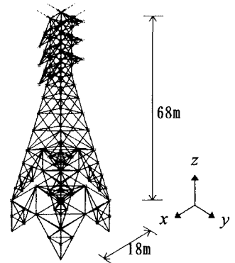
図-1 3次元トラス
