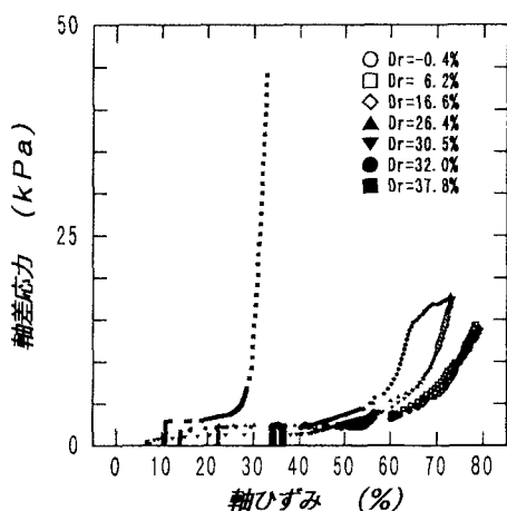
図-1 q \sim \varepsilon 関係
