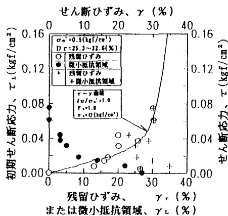
図-5 初期せん断応力～微小抵抗領域関係図 [ \sigma'_o = 0.5(\text{kgf/cm}^2) ]
