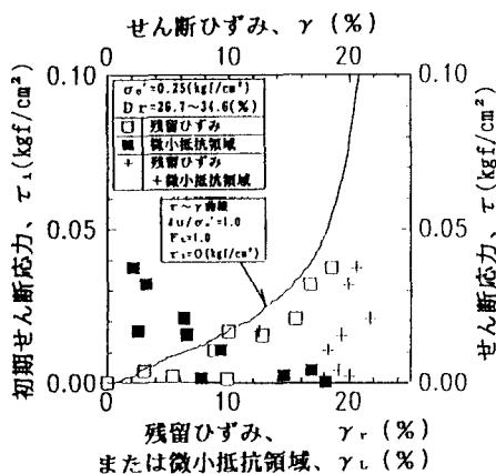
図-4 初期せん断応力～微小抵抗領域関係図 [ \sigma'_o = 0.25(\text{kgf/cm}^2) ]
