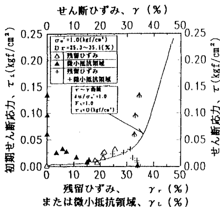
図-6 初期せん断応力～微小抵抗領域関係図 [ \sigma'_o = 1.0(\text{kgf/cm}^2) ]
