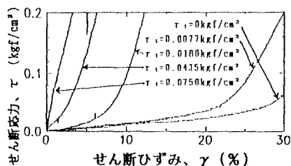
図-2 液状化後の応力 \tau ～ひずみ \gamma 関係拡大図
