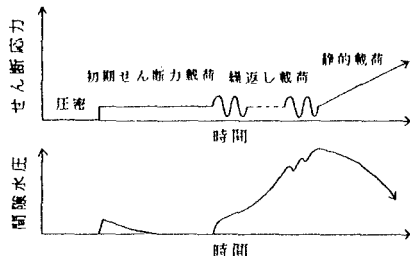
図-1 载荷パターン
