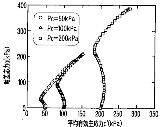
図-5 有効応力経路
